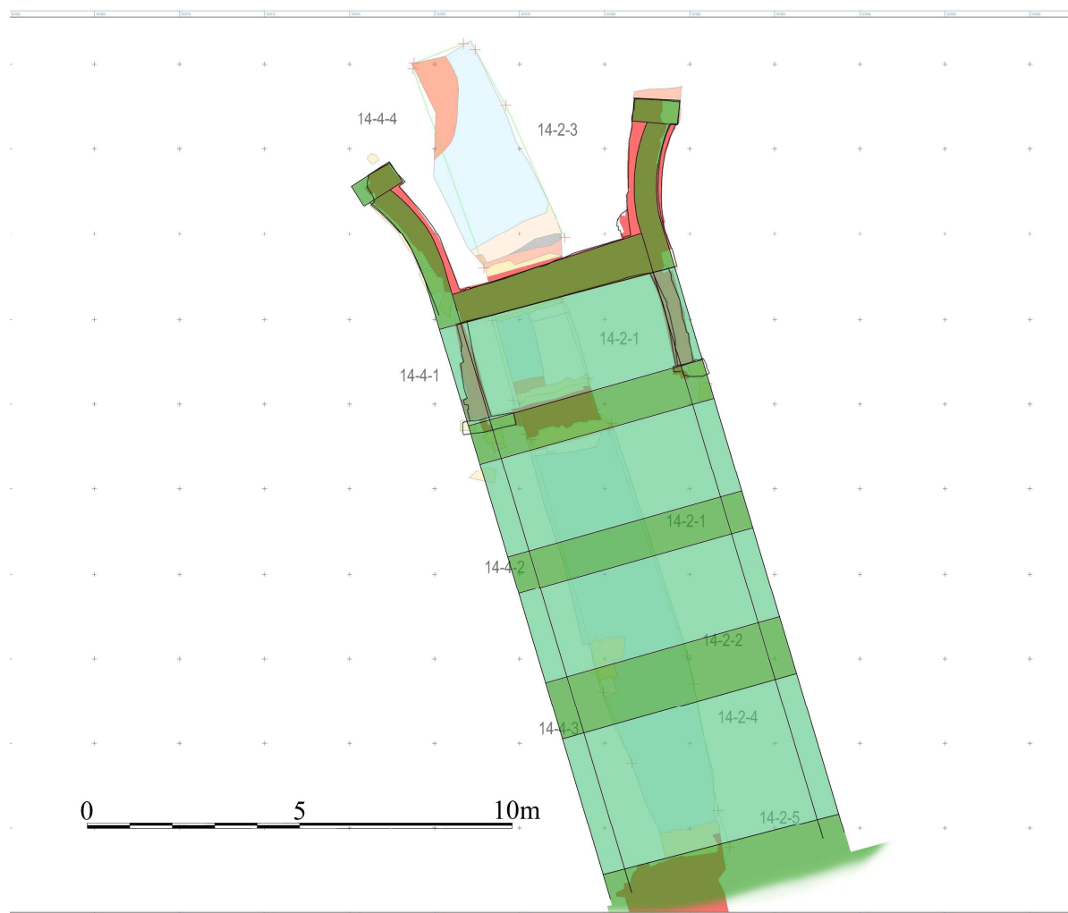
003. Plattegrond van de brug samengesteld met de plattegrond van RAAP (de rood, geel en blauw gekleurde delen), de contour van het bruggenhoofd op basis van de gegevens van Hagens (de zwarte lijnen ter plaatse van het bruggenhoofd aan de landzijde) en de schematische uitwerking van de opmeting van Adolph Mulder (donkergroen voor de bruggenhoofden en brugpijlers en lichter groen voor de gewelven). Uit de projectie is af te leiden dat alle drie opmetingen vrijwel volledig met elkaar overeenkomen.
