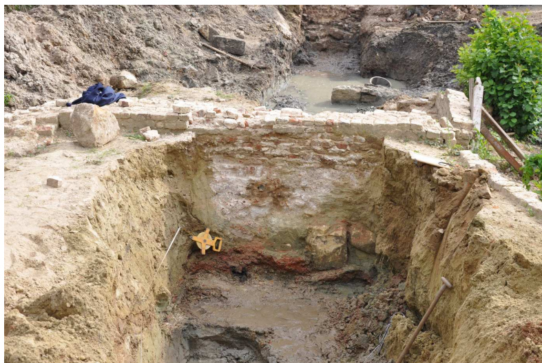
008. Detail van de binnenzijde van het bruggenhoofd. Het metselwerk is hier voorzien van een zeer harde laag mortel. Het metselwerk zelf is onregelmatig en slordig uitgevoerd.
